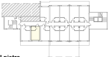
Rzut II piętra
